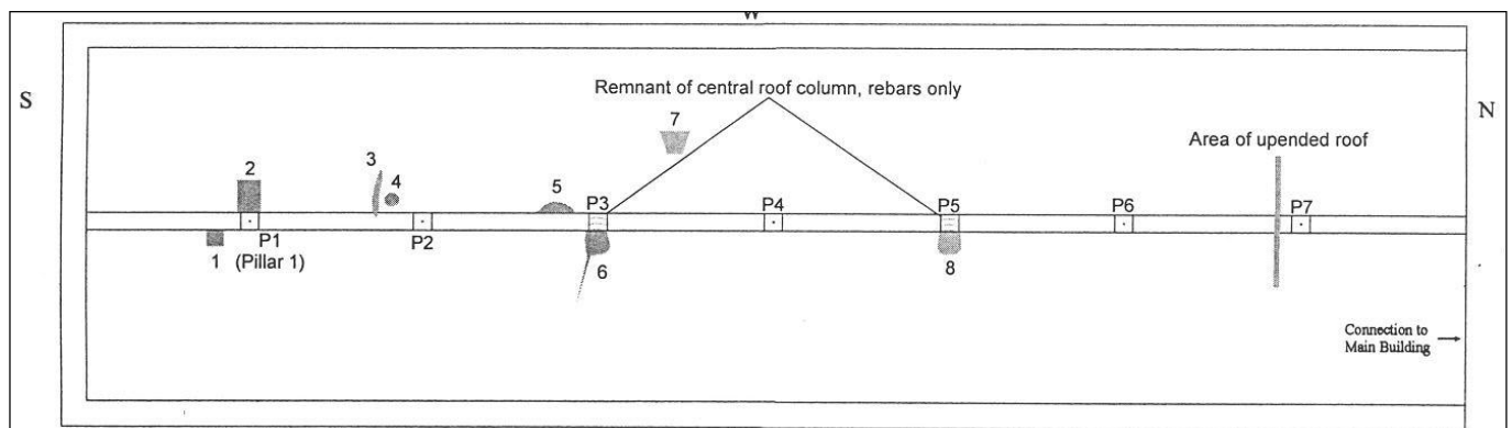
Schematische Zeichnung der Decke des Leichenkeller 1 von Krematorium II in Auschwitz-Birkenau von Charles Provan in »No Holes? No Holocaust« abgebildet, unpaginiert (S. 36).
